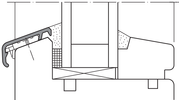
Einbaubeispiel FA 21 Installation example
